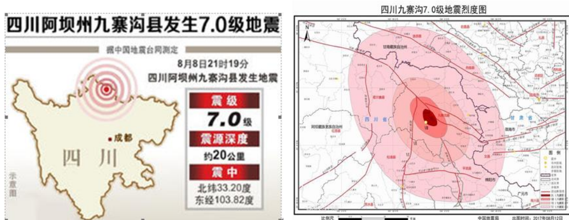
图1 九寨沟7.0级地震示意及剧烈度图
